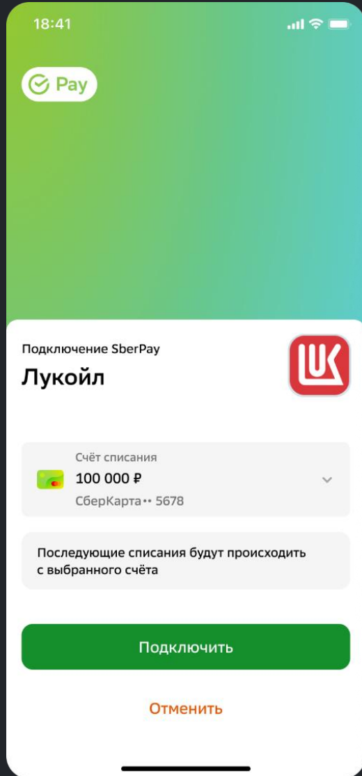
Экран оплаты
