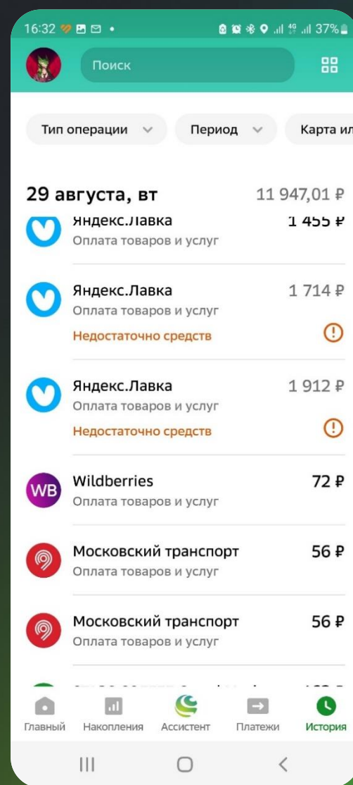
Список операций
