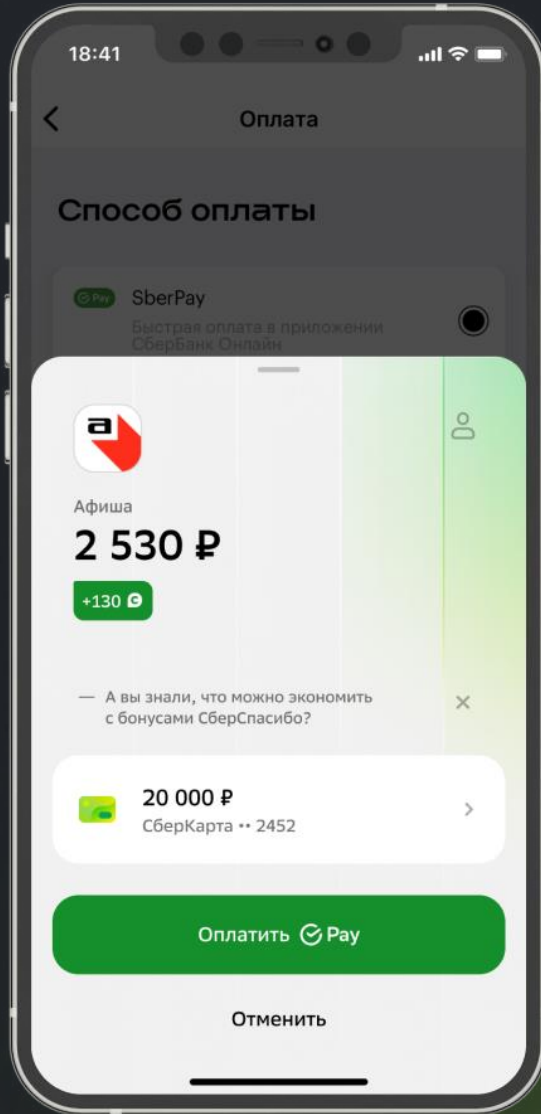
SberPay SDK
